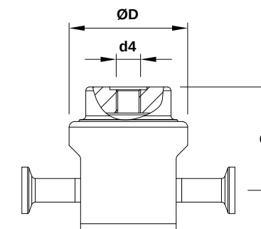
Optional dome-loading
