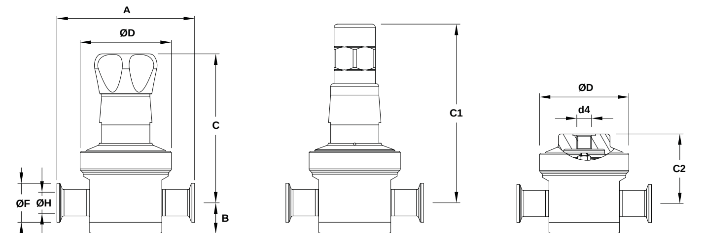
Optional top cap
