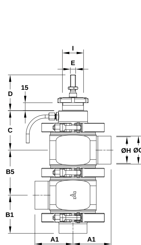
V928MV
