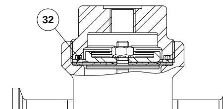
Optional dome-loading
