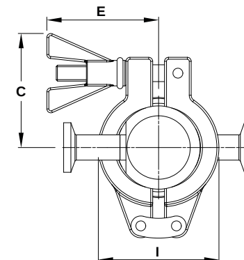
TSS6A
